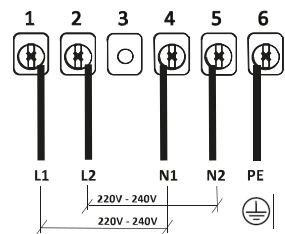
NL 230V / 400V 2N ~
