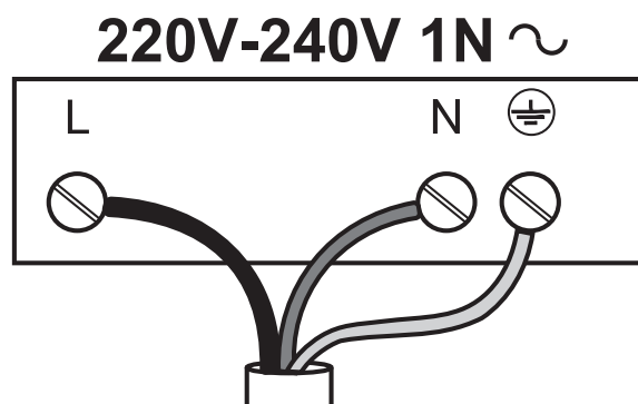
Esquema de ligação
