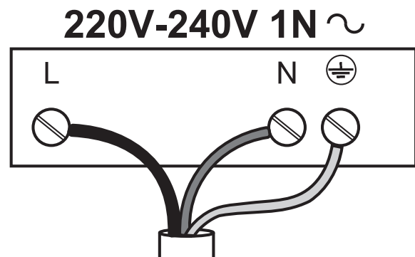
Schema de conexiune
