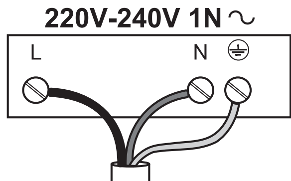
Шема прикључивања
