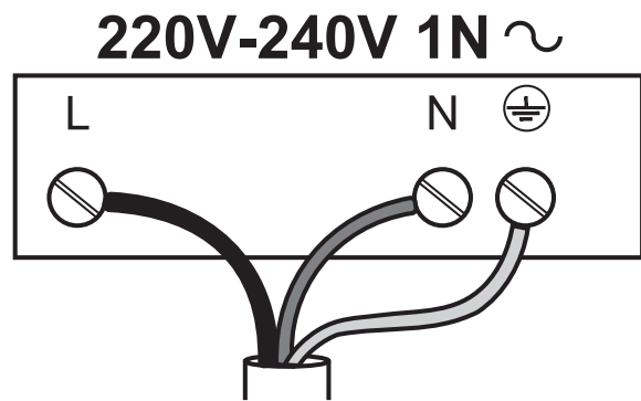
Jungimo schema
