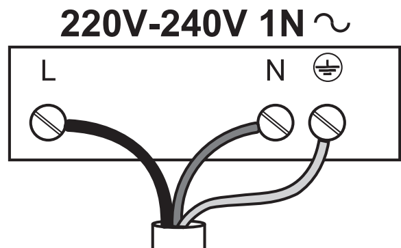
Esquema de conexión
