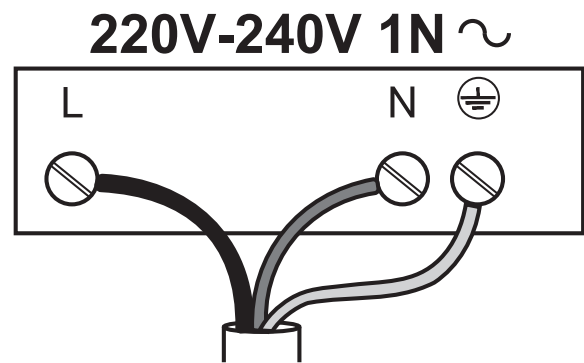
Схема на свързване
