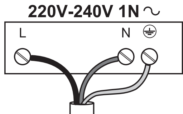
Schemat połączeń
