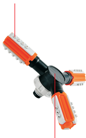
Główna część obrotowej dyszy (średnica gwintu około 25mm)
