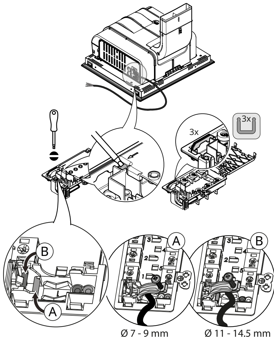
Schemat Połączeń Kablowych
